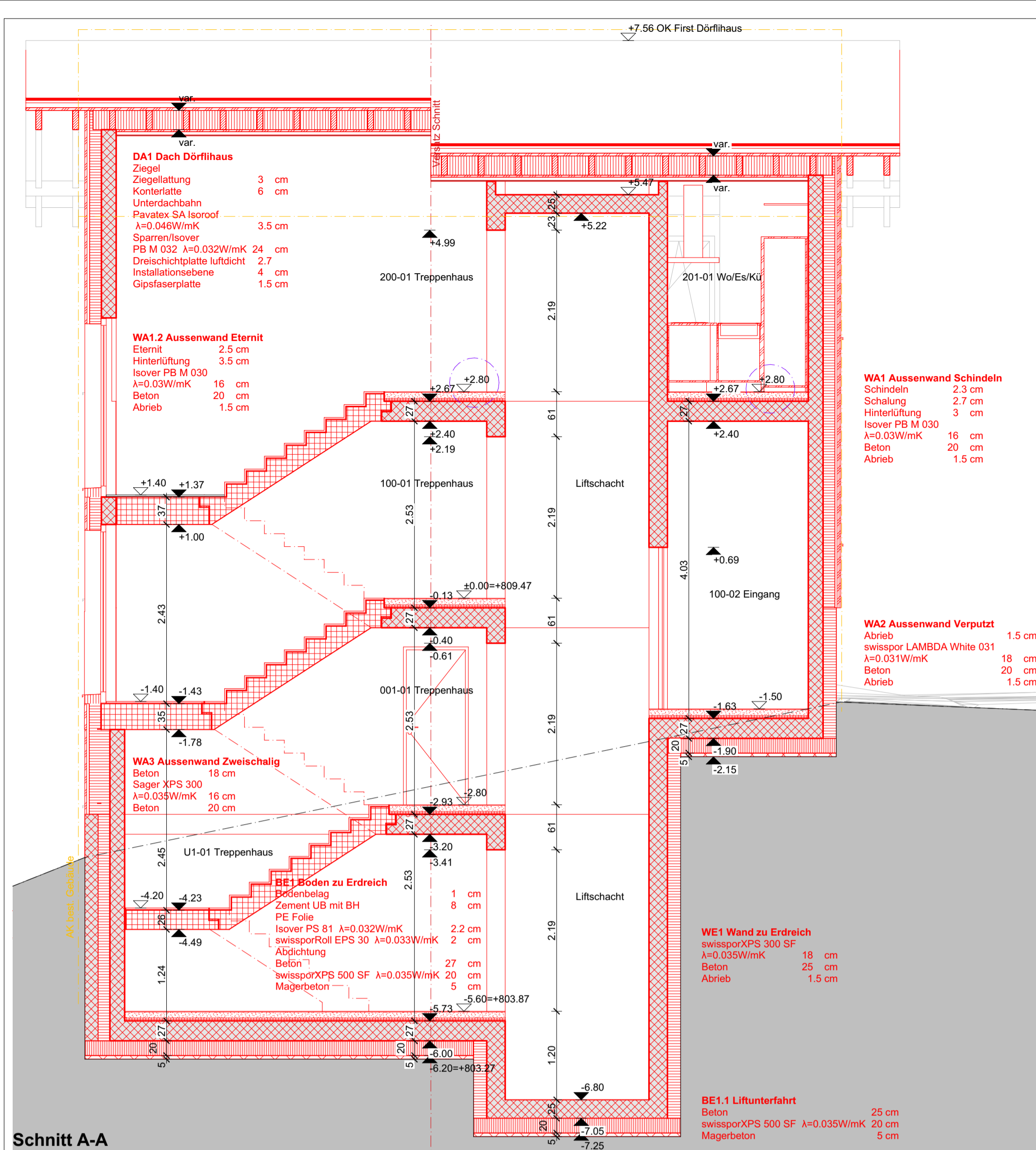
Schnitt A-A
