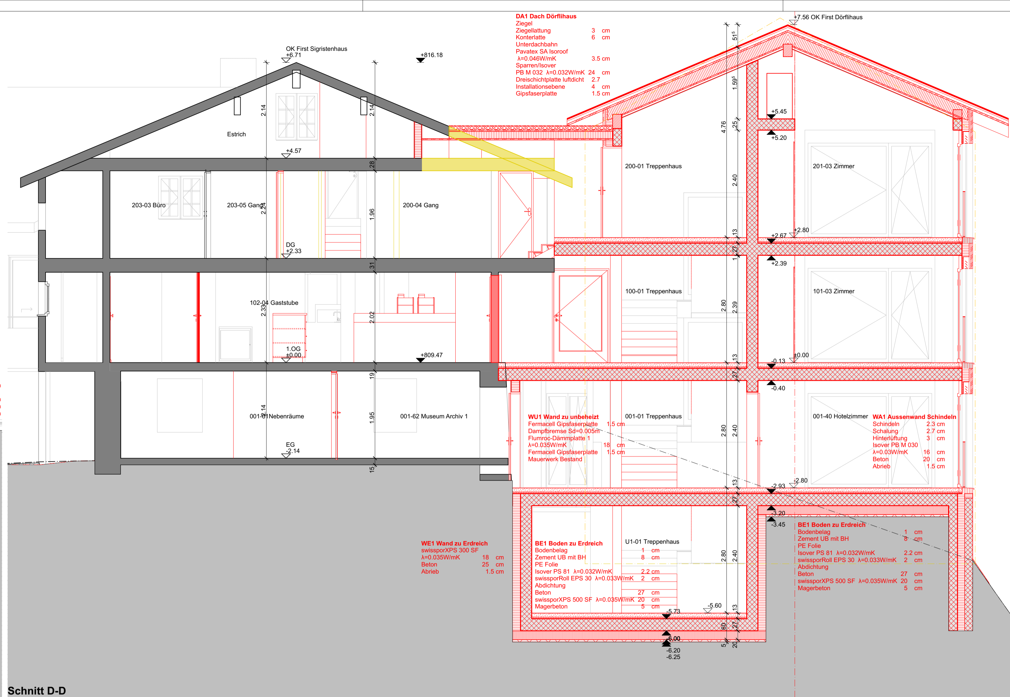
Schnitt D-D
